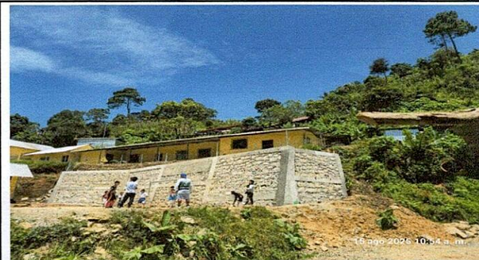
Foto 4: Observación de muro de contención con el avance del 95%
