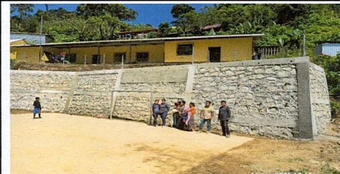
Foto 6: Finalización y entrega de proyecto de remozamiento: muro de contención y cuneta
